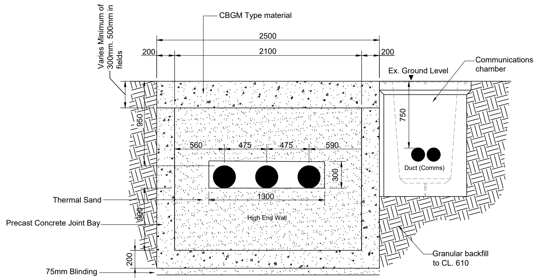
Section A-A
