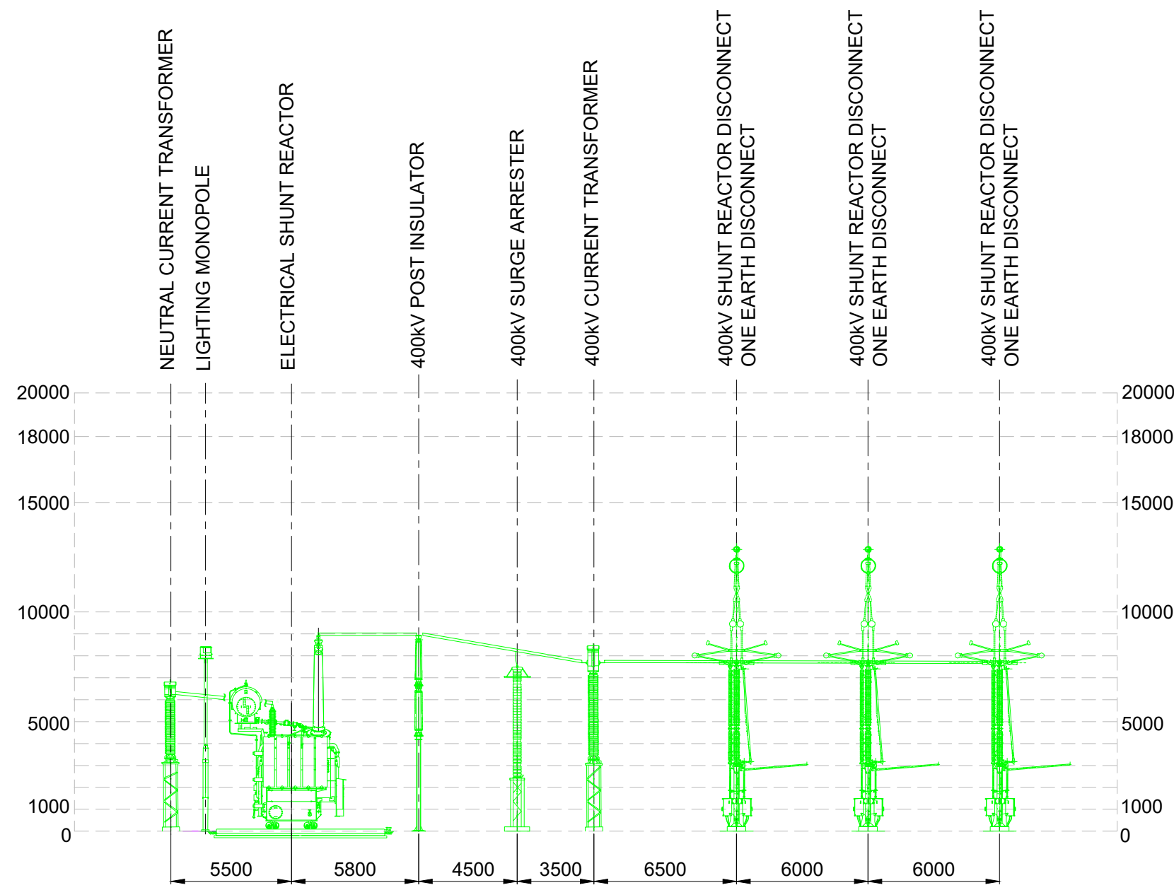
SECTION A-A SCALE : 1:250
